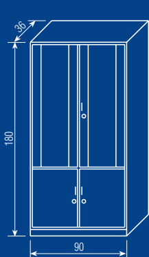
SS2-90 segment częściowo oszkłony
