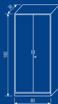
S2-80 szafa na dokumenty
