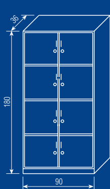
S8-90 segment z szafkami osobistymi
