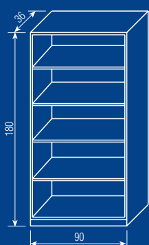
R-90 regał otwarty
