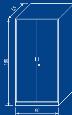
SU-90 szafa ubraniowa
