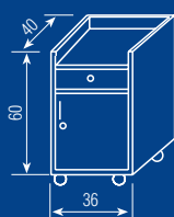
D-1 dostawka biurka zamykana
