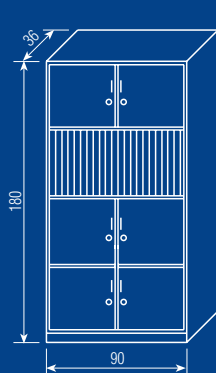
SD-90 segment z przegrodami na dzienniki klasowe
