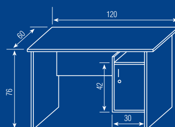
B biurko nauczycielskie z szafką
